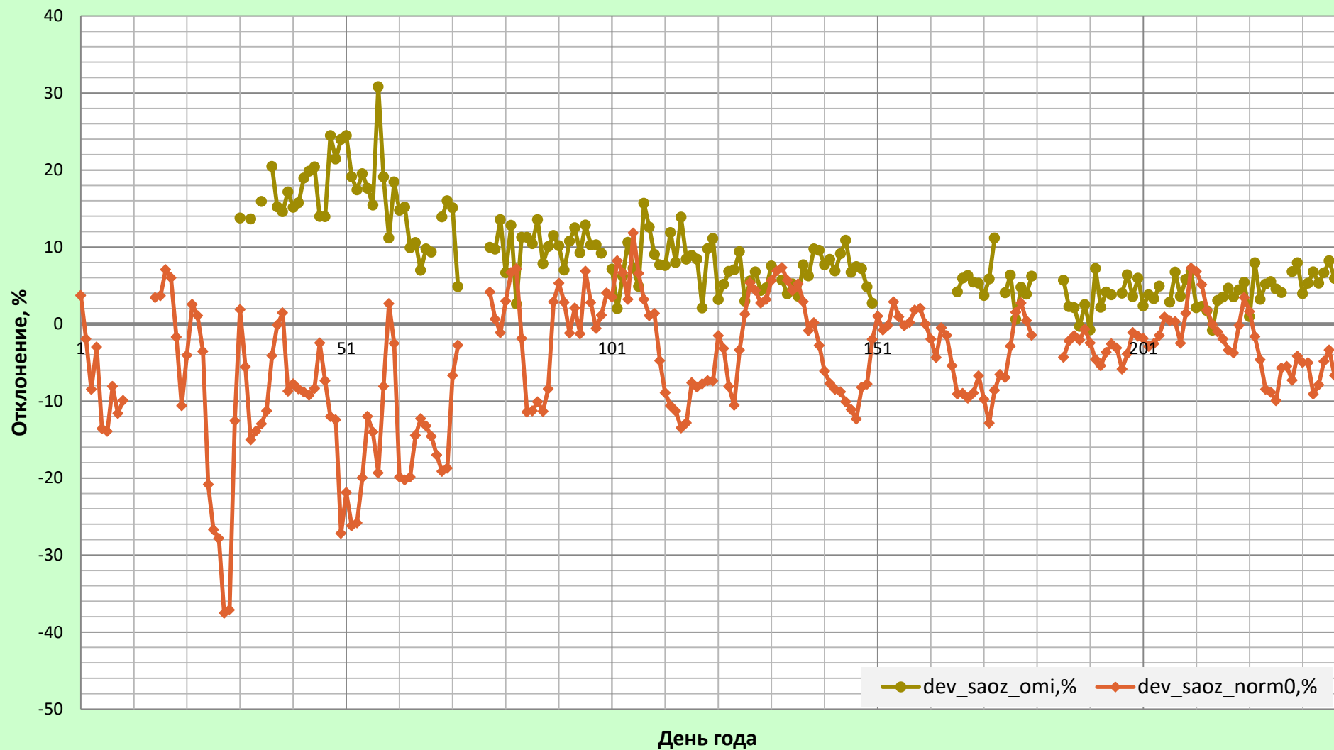
Отклонения (%) данных наземных измерений OCO (Mini-SAOZ) от данных спутниковых измерений OCO (OMI,NASA) и отклонение наземных измерений (Mini-SAOZ) от климатических норм для ст.Салехард, 1 января - 24 августа 2016 года.
