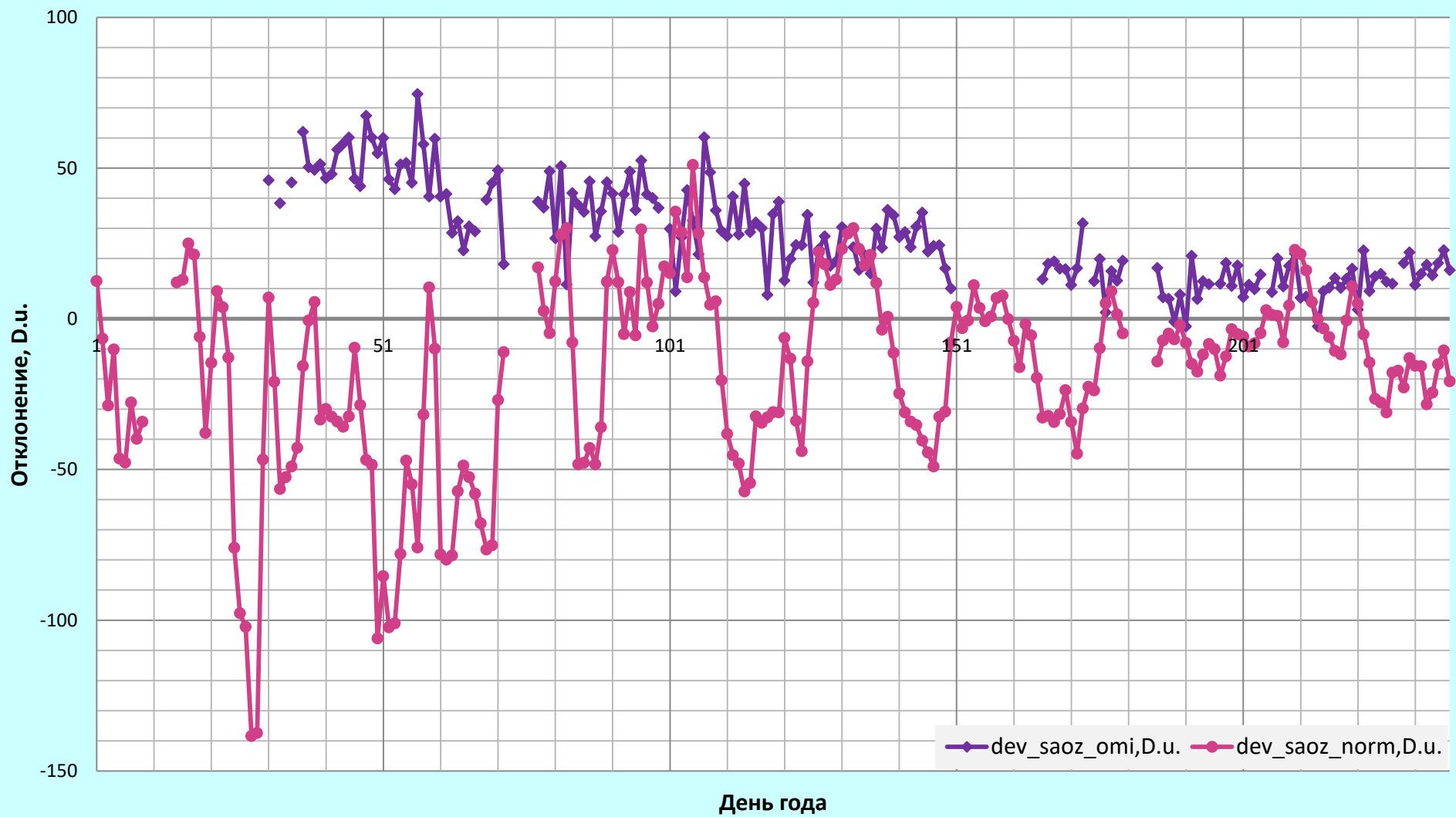
Абсолютные отклонения (D.u.) данных наземных измерений OCO (Mini-SAOZ) от данных спутниковых измерений OCO (OMI,NASA) и отклонение наземных измерений (Mini-SAOZ) от климатических норм для ст.Салехард, 1 января - 24 августа 2016 года.
